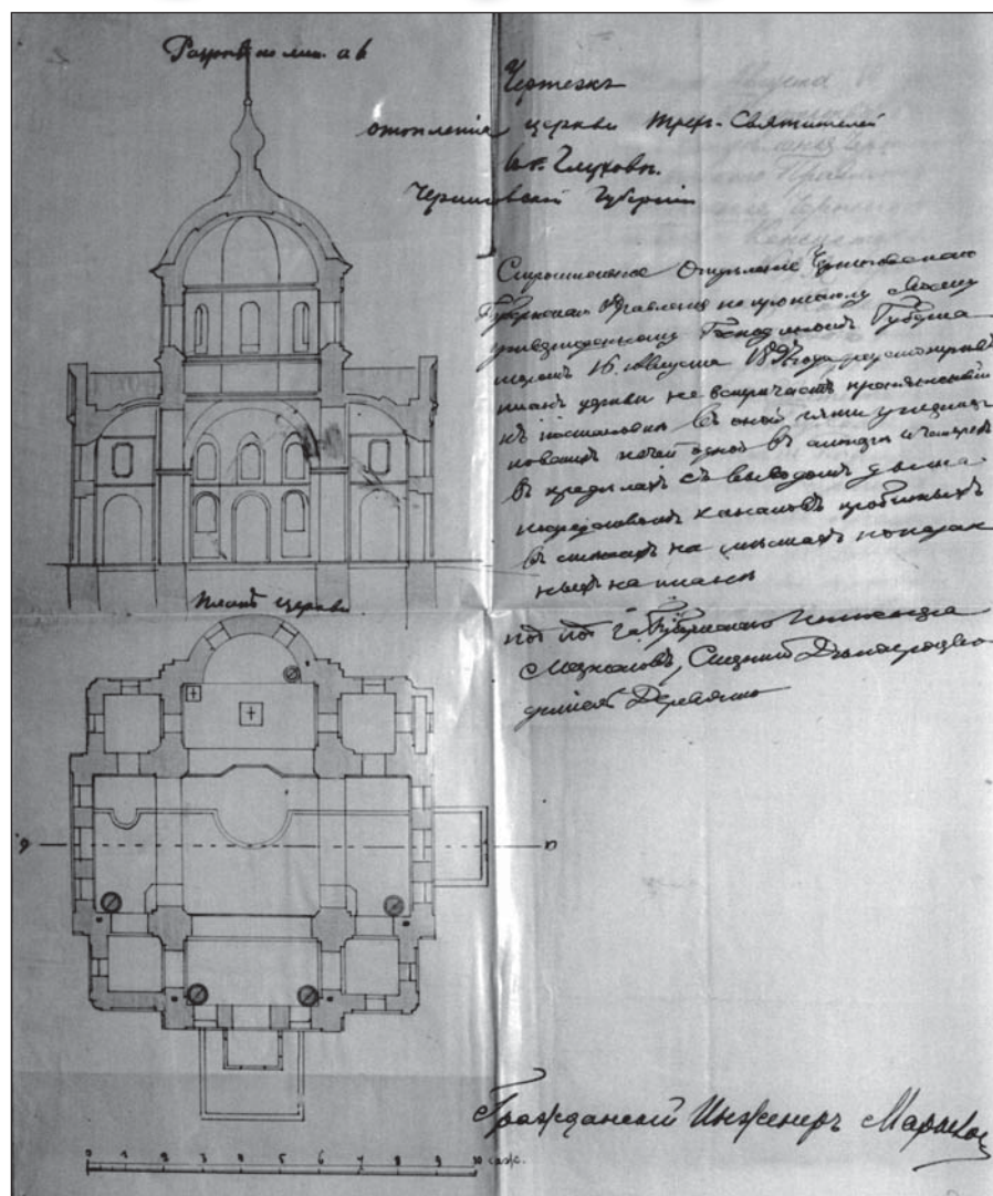
Креслення улаштування опалення Трьохсвятської церкви (1897 р.)
