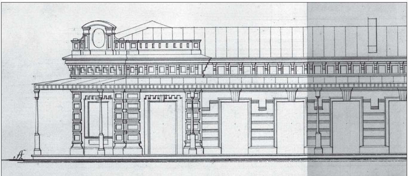
Фрагмент проекту улаштування мурованих торгових лавок у Глухові. ДАЧО, ф. 127, оп. 10, спр. 613
