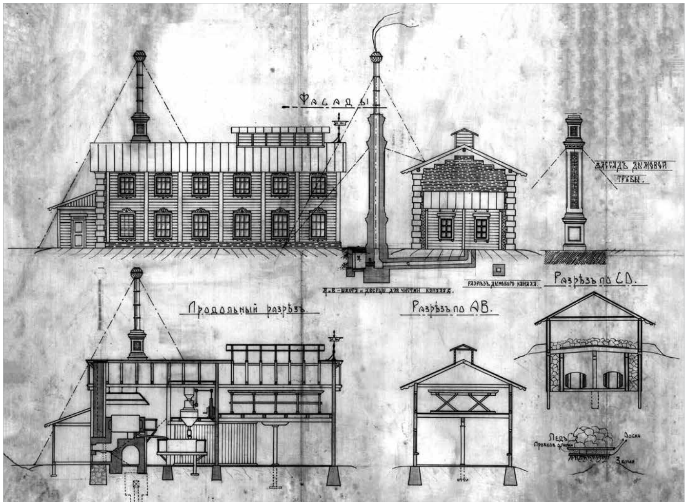
Фрагмент проекту пивоварного заводу у Глухові австрійських підданих А.С. Бештака та Б.І. Блажека
