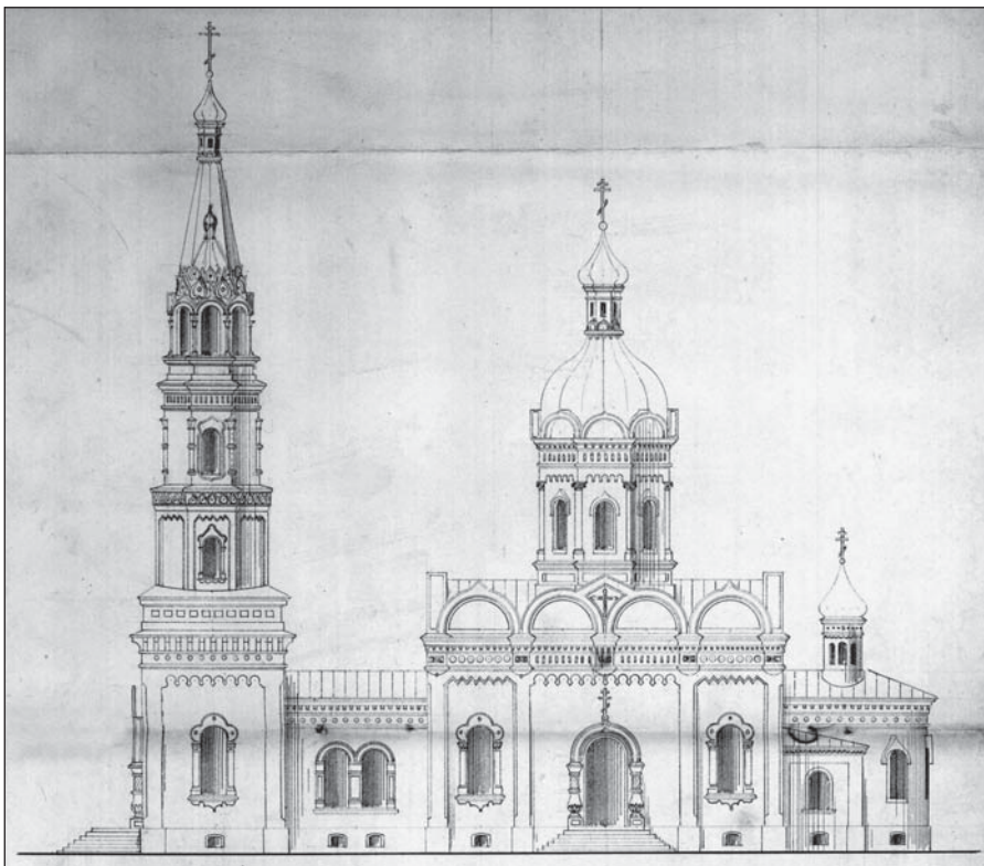
Кресленик фасаду церкви св. Миколая в с. Есмань. 1864 р.
