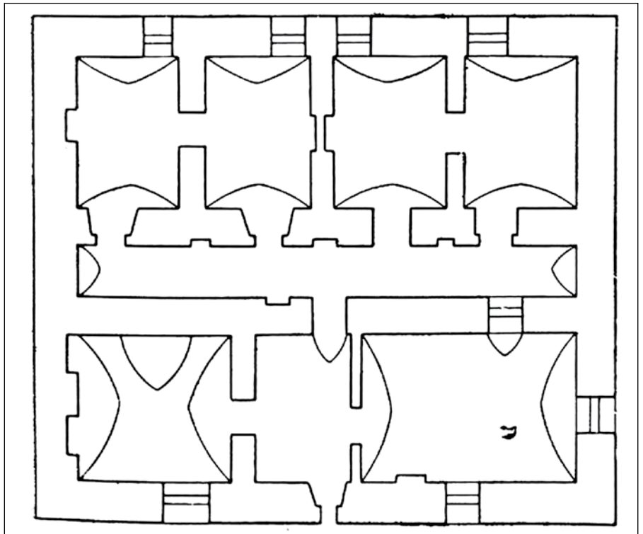
Житловий будинок у Глухові (XVIII ст.). План першого поверху
