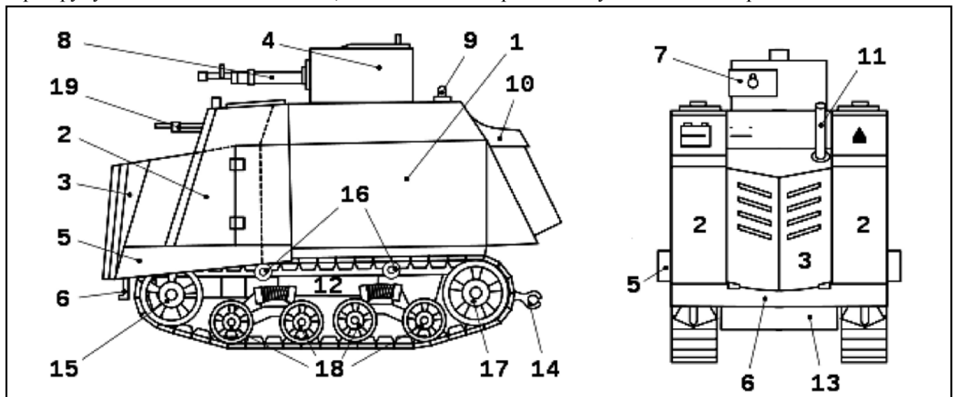
Рис. 1. Компонувальна схема танка «НИ»: 1. корпус, 2. бокові частини корпусу, 3. моторний відсік, 4. башта, 5. грязеві щитки, 6. бронещиток ходової частини, 7. маска кулемета, 8. кулемет ДШК, 9. монтажний рим, 10. інструментальний ящик, 11. вихлопна труба, 12. бокові консолі рами, 13. передній лист рами, 14. буксировочний гак, 15. натяжне колесо, 16. підтримуючий ролик, 17. ведуче колесо, 18. каток каретки, 19. кулемет ДТ.
