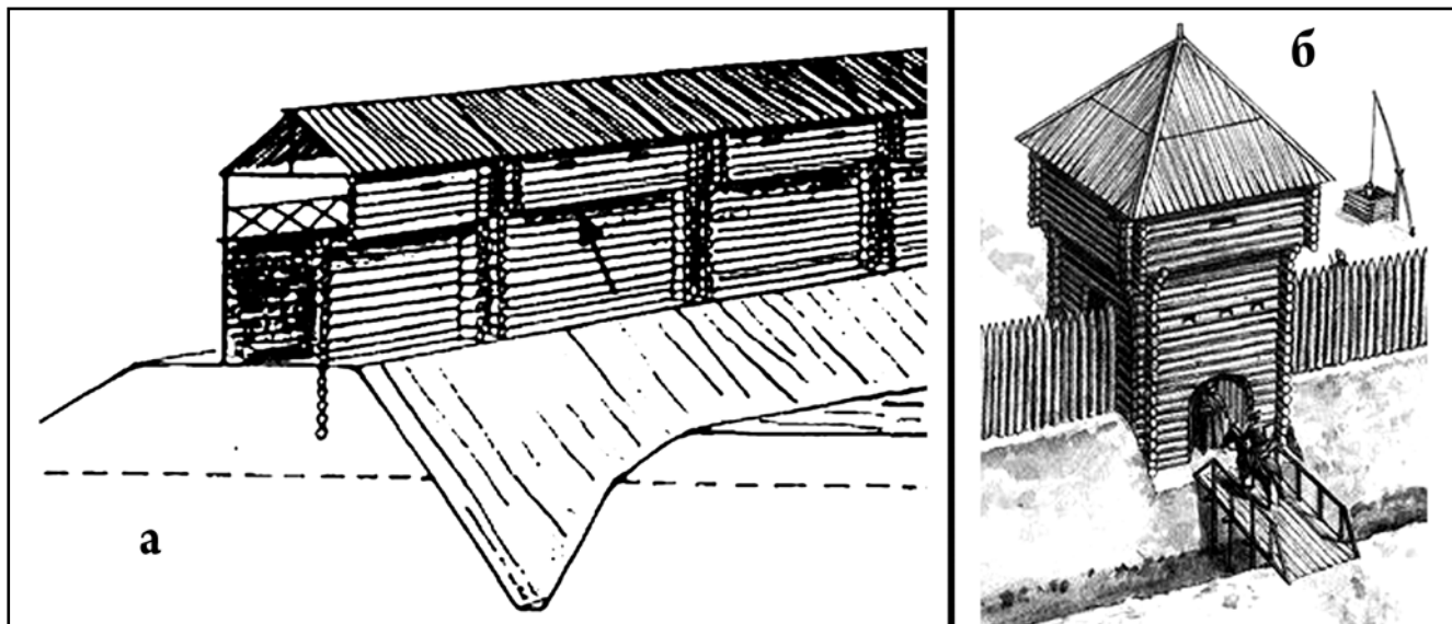
Рис. 2. Укріплення активної оборони
