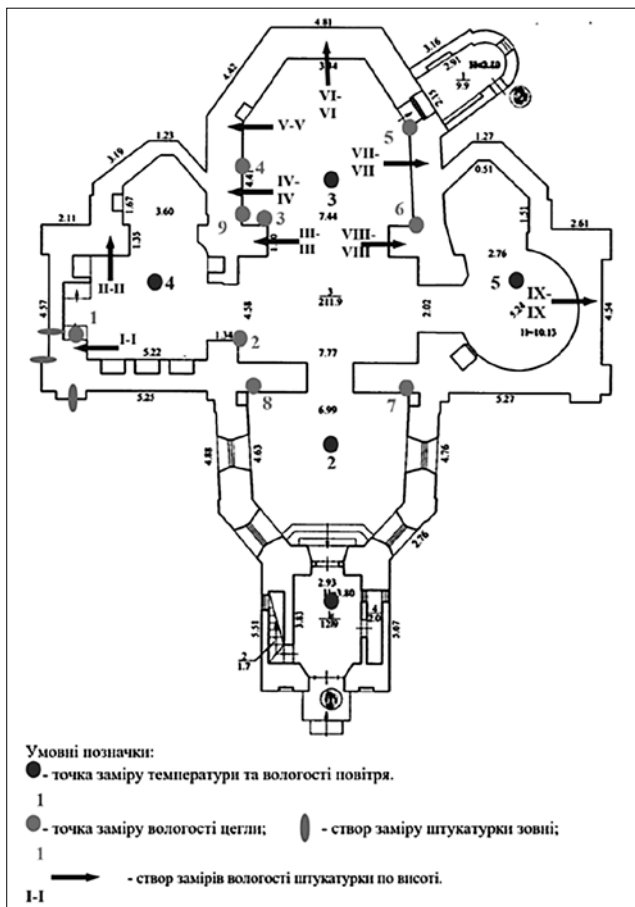
Рис. 3. План-схема розташування точок замірів вмісту вологи (вагової вологості) у будівельних матеріалах (цегла, будівельні розчини) у церкві Спаса на Берестові.
