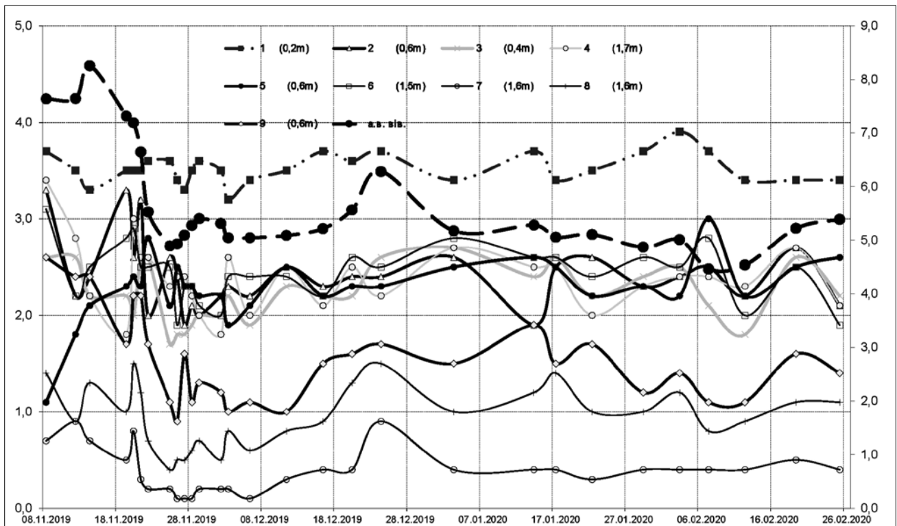
Рис. 5. Графіки коливань вагової вологості цегли та абсолютної вологості повітря в інтер'єрі церкви (у % по правій шкалі), листопад 2019 – лютий 2020
