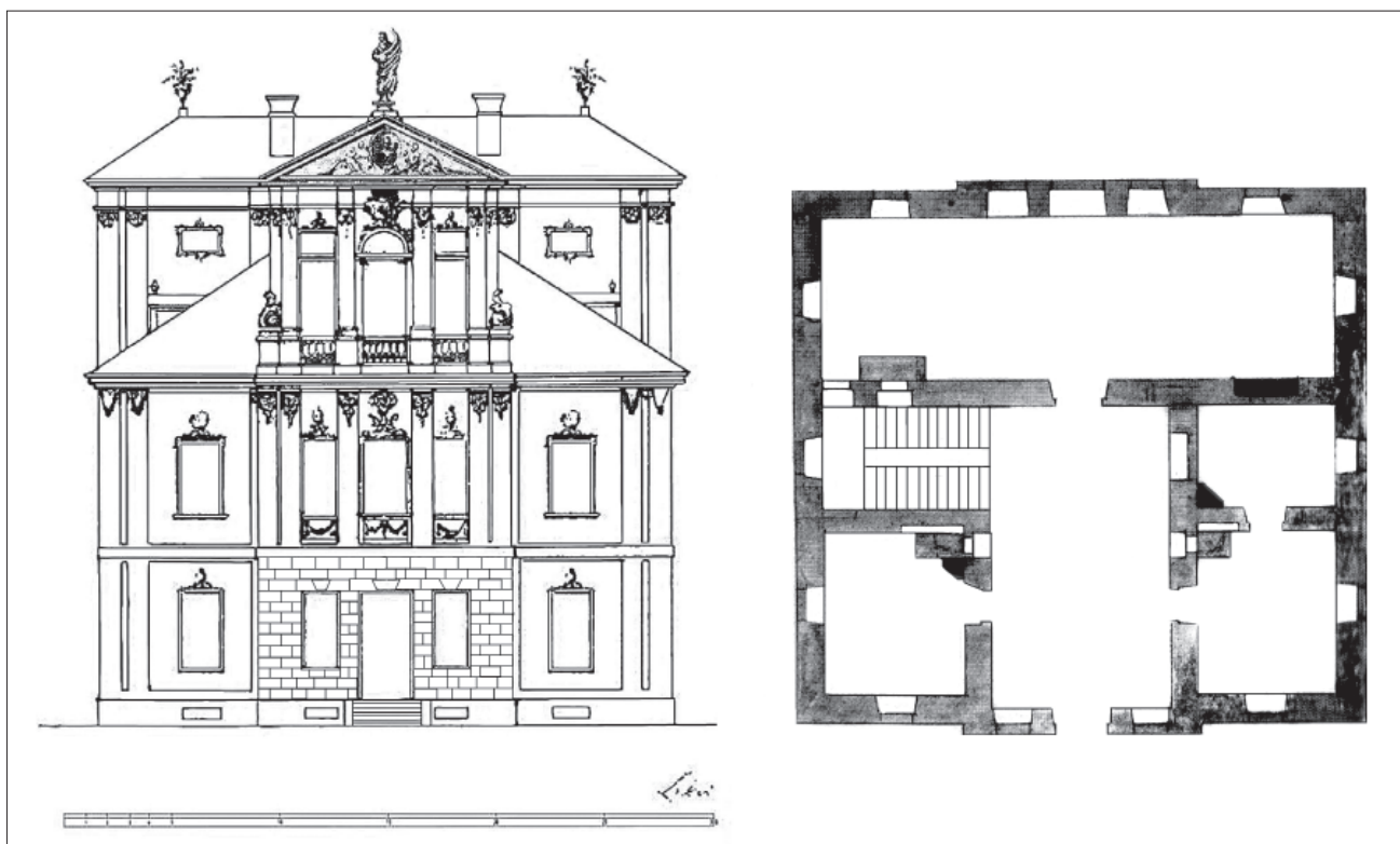
Рис. 15. Кресленики Т. Гамерена чільного фасаду з ризалітом та плану палацу Котовських у Варшаві 1684 р. Посилання 36.
